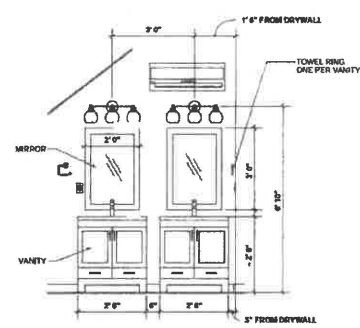
4 BATHROOM ELEVATION SCALE: 1/8" = 1'-0"
