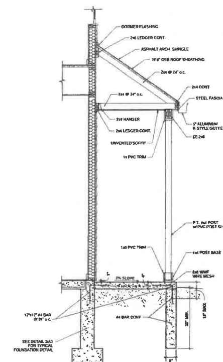
6 PORCH SECTION SCALE: 3/8" = 1'-0"
